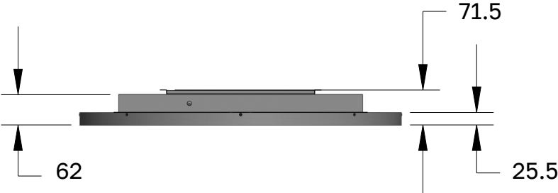
СХЕМА ДИСПЛЕЯ (ВИД СВЕРХУ)
