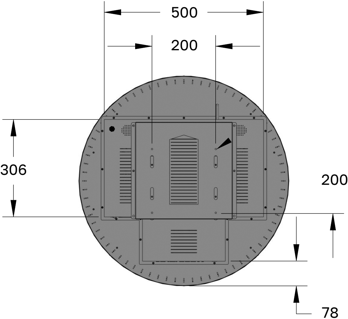
СХЕМА ДИСПЛЕЯ (ВИД СЗАДИ)
